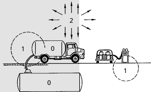
Beispiel für Zonenbestimmung in explosionsgefährdeten Bereichen Example for zone localisation explosion-endangered area
