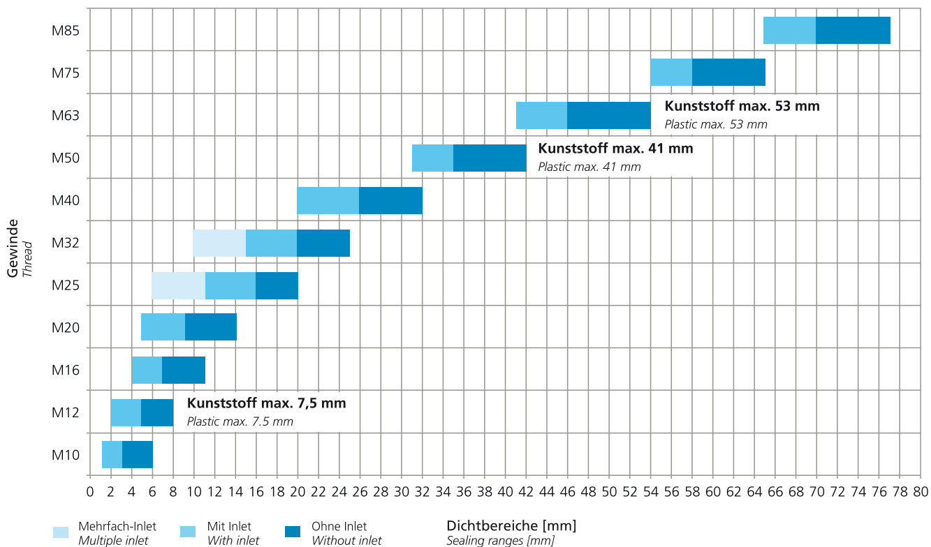
Dichtbereiche der blueglobe Sealing ranges of blueglobe
