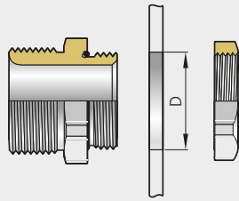
Abb. 1 – Durchgangsbohrung Fig. 1 – Through-hole
