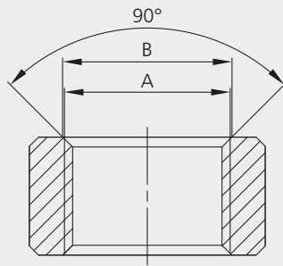
Abb. 2 – Gewindebohrung Fig. 2 – Threaded hole
