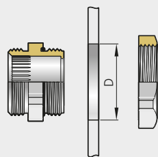
Abb. 1 – Durchgangsbohrung Fig. 1 – Through-hole
